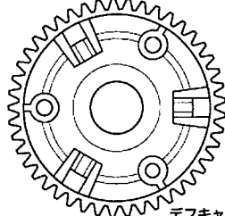
GB3 デフキャリア Differential gear case Differentialgehäuse Carter de différentiel X1
